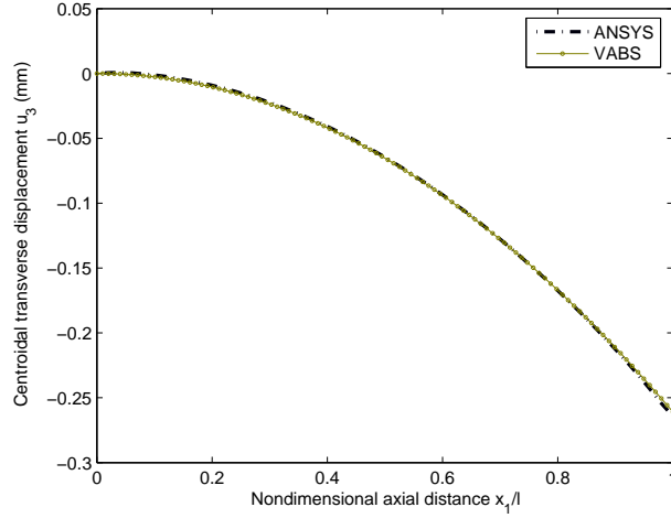
Fig. 2. Transverse displacement
